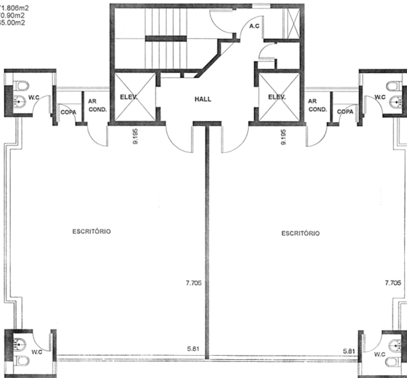
PLANTA PAV. TIPO
