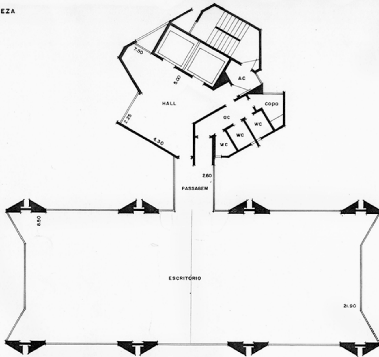
PLANTA PAV. TIPO
