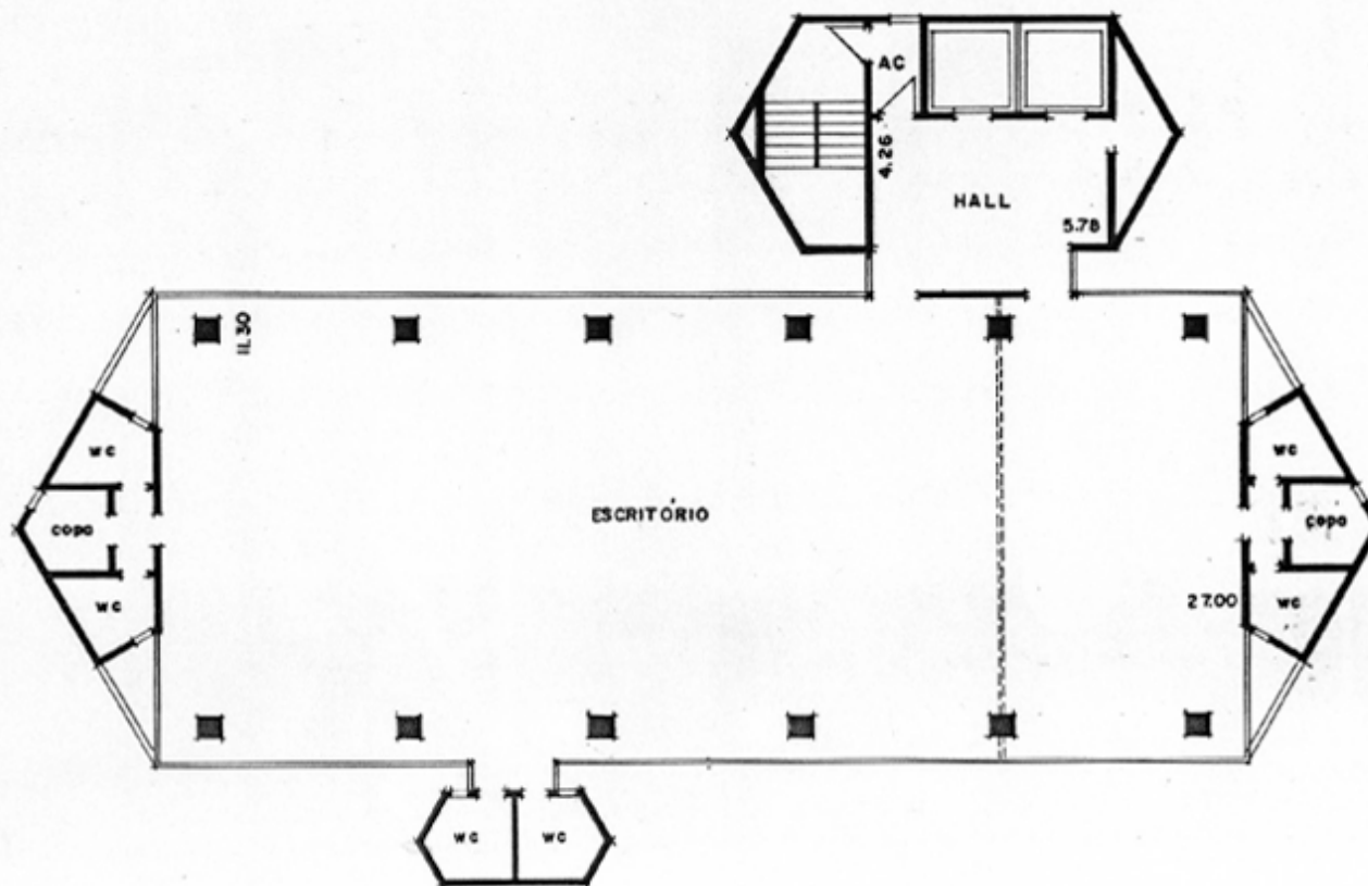
PLANTA PAV. TIPO
