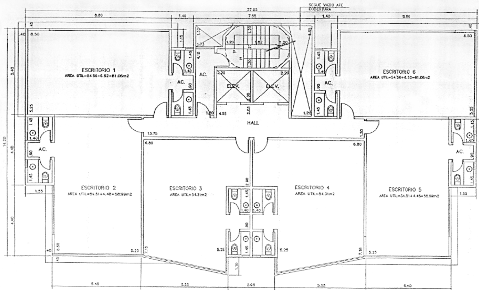
PLANTA PAV. TIPO
