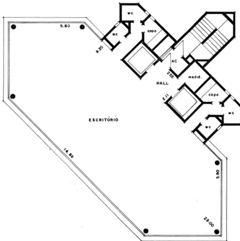
PLANTA PAV. TIPO
